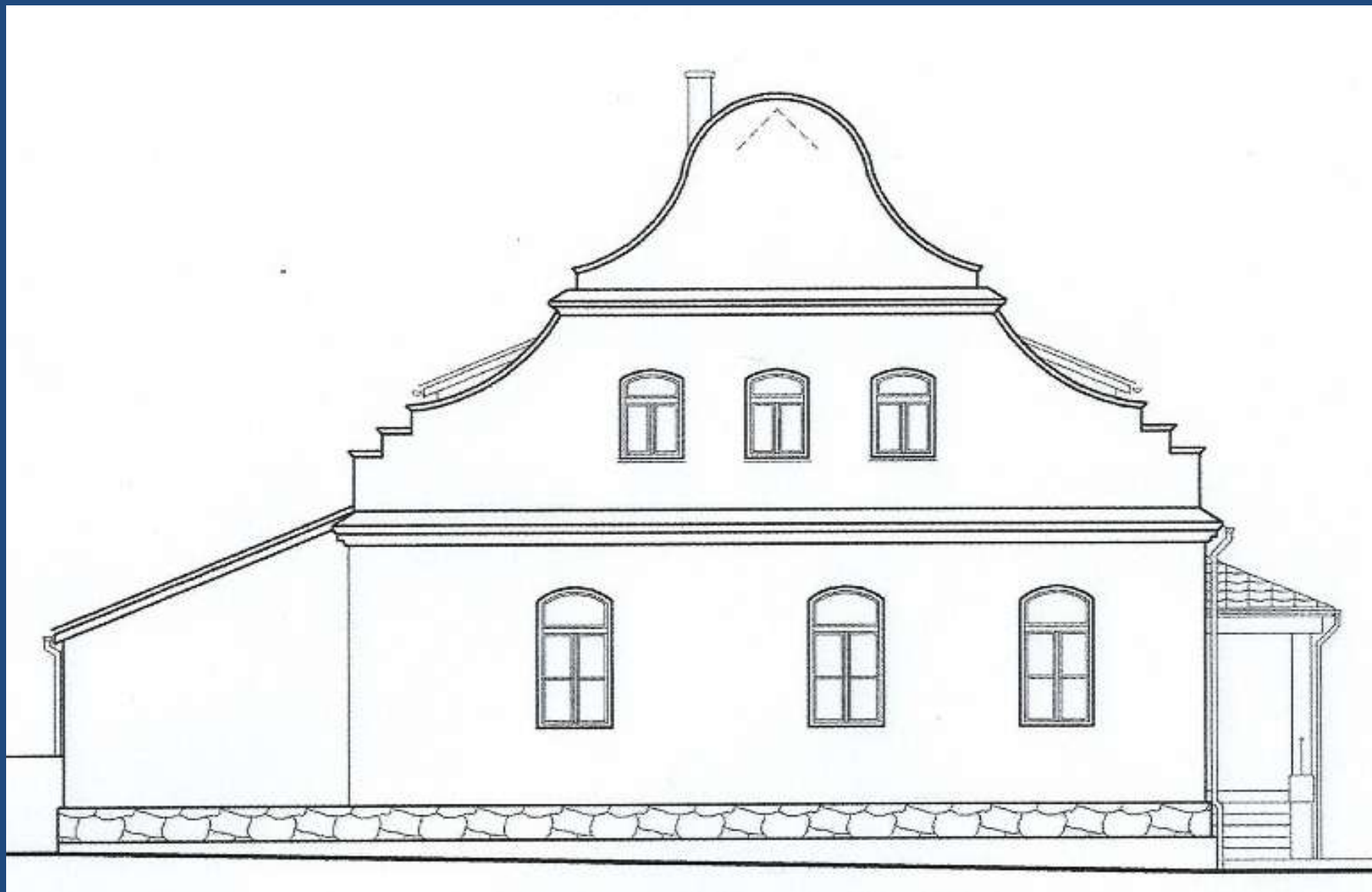
Severní pohled
