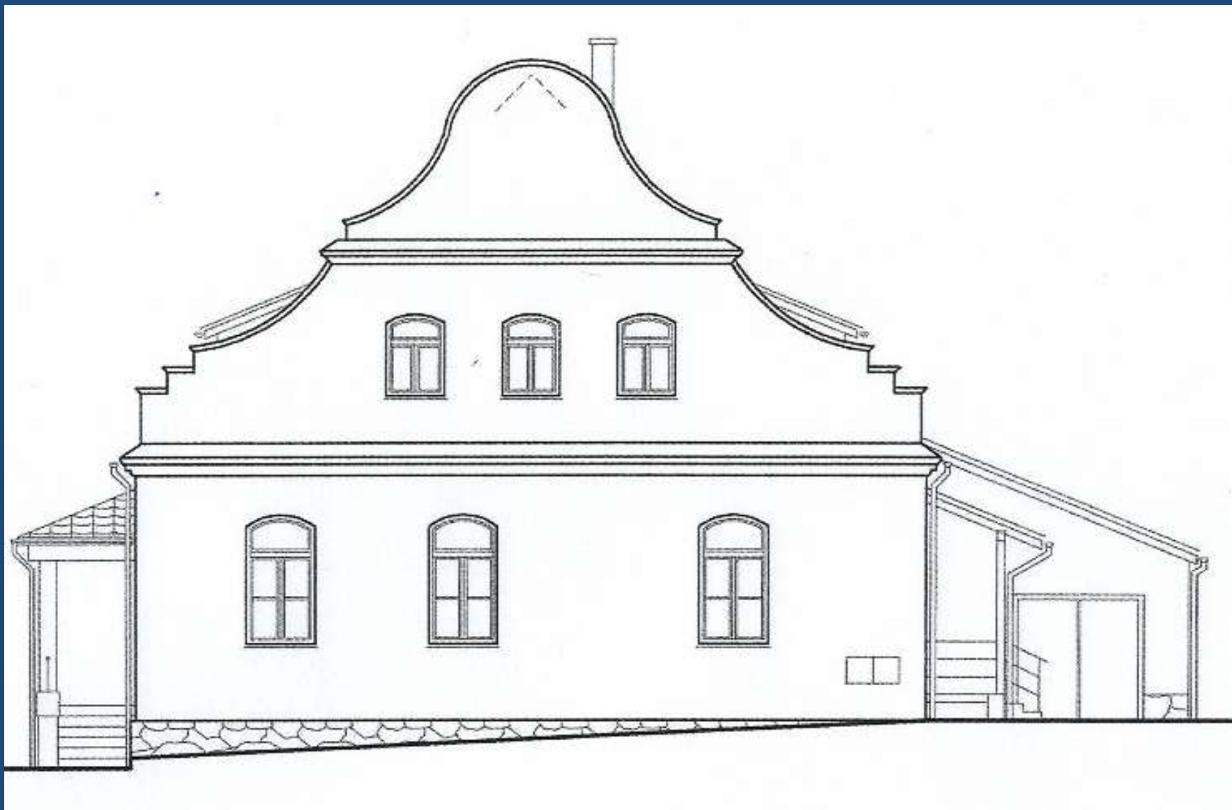
Jižní pohled
